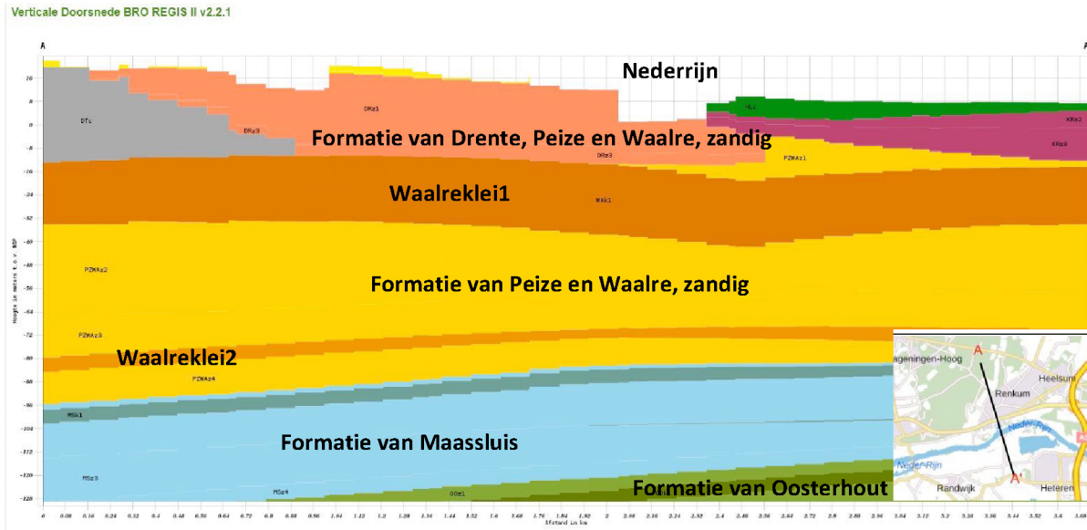
Figuur 2-5: Geohydrologische dwarsdoorsnede van noord naar zuid over Renkums Beekdal, Parencu en Betuwe (Bron: REGIS II.2 uit DinoLoket)
