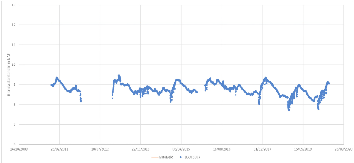
Figuur 3-19: Gemeten grondwaterstand in peilbuis B39F3007 (Bron: DinoLoket)
