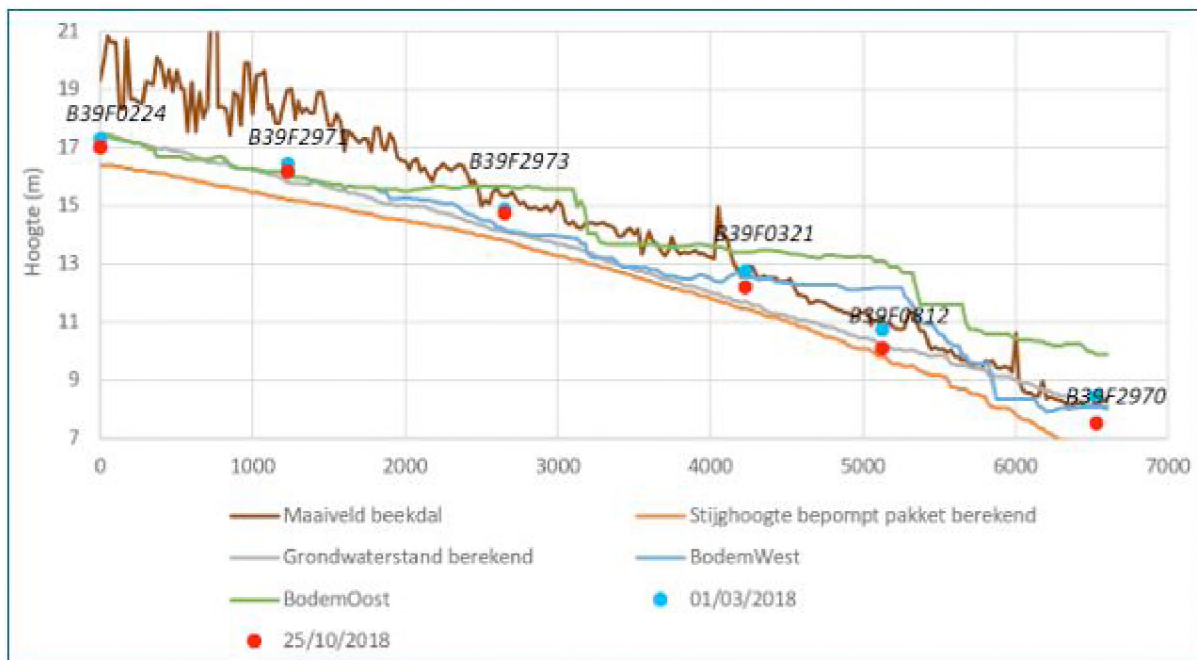
Figuur 3-5: Lengteprofiel Renkums beekdal. De punten geven gemeten grondwaterstanden weer. De lijnen berekende stijghoogtes in de huidige situatie
