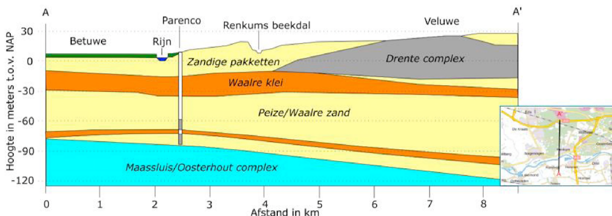
Figuur 2-4: Doorsnede zuid-noord langs de winning van SK Parencó (o.b.v. REGIS II v2.2)
