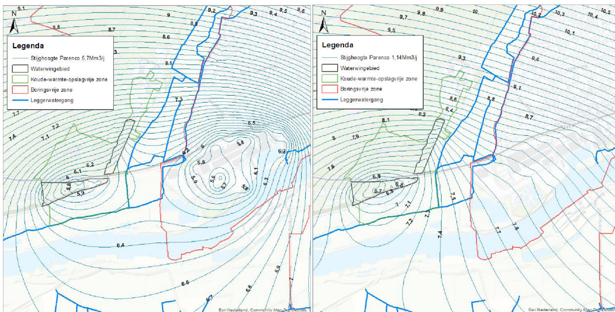
Figuur 3-17: Berekende isohypsen in het bebompte pakket bij een winning van 5,7 Mm 3 /jaar bij SK Parencó (vergunde situatie, rechts) en 1,14 Mm 3 /jaar SK Parencó rechts). De waterscheiding ligt in de figuur links vlak naast het terrein van SK Parencó
